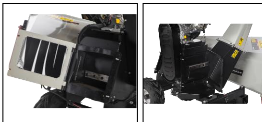
Klappbarer Einfüll- und Auswurftrichter
