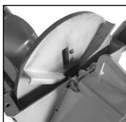
Scheibenrad mit Flügeln und Messer
